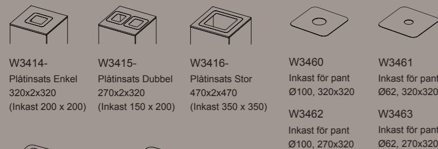
W3440 Inkast enkel med täcklock Inkast 200 x 200 W3441 Inkast dubbel med täcklock till dubbelt inkast Inkast 150 x 200
