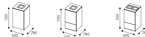
W3211 Hel dörr för rullkärl 190 l W3212 Dörr ovan till för 1x90 l kärl och lādudrag undertill * W3213 Dörr ovan till för 2x60 l kärl och lādudrag undertill *
