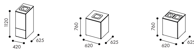
W3114 Dörr ovan till för 1x60 l kärl och lādudrag undertill ** W3115 Låg modul med hel dörr för 1x90 l kärl W3116 Låg modul med hel dörr för 2x60 l kärl
