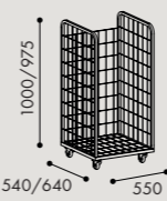
W0101 Vagn för kartonger M W0103 Sidor till vagn M W0102 Vagn för kartonger L W0104 Sidor till vagn L
