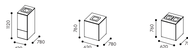
W3214 Dörr ovan till för 1x60 l kärl och lādudrag undertill ** W3215 Låg modul med hel dörr för 1x90 l kärl W3216 Låg modul med hel dörr för 2x60 l kärl
