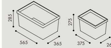
W0016 Kärl 42 liter, inkl 2 skiljeväggar
