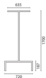
Dubbelstativ
