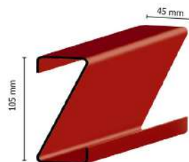
Utförande: Z105-20
