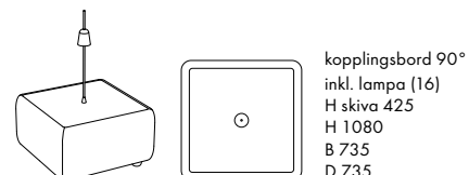
kopplingsbord 90° inkl. el (15) H 425 B 735 D 735
