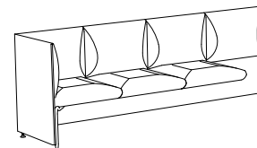
SA830 hörnkoppling (19) H 850 SH 450 B 2555 D 665
