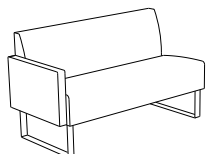
SA610/ SA620/ SA630 H 795 SH 450 B 620/1370/1770 D 630
