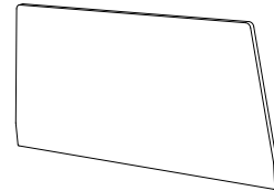
SA350 kupévägg mellan (17) H 1315 B 2620 D 45
