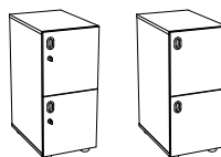
förvaringskåp (25) H 1000 B 400 D 600
