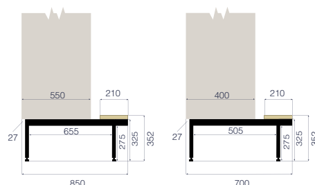
Bänkstativ med sits av björklaminat
