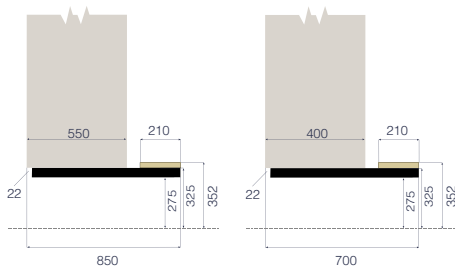
Bänkkonsol med sits av björklaminat
