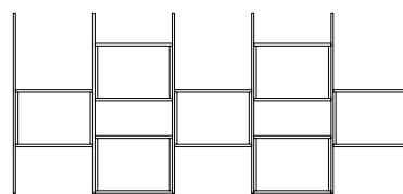
5 dubbelsidiga sektioner = 7 stålramar
