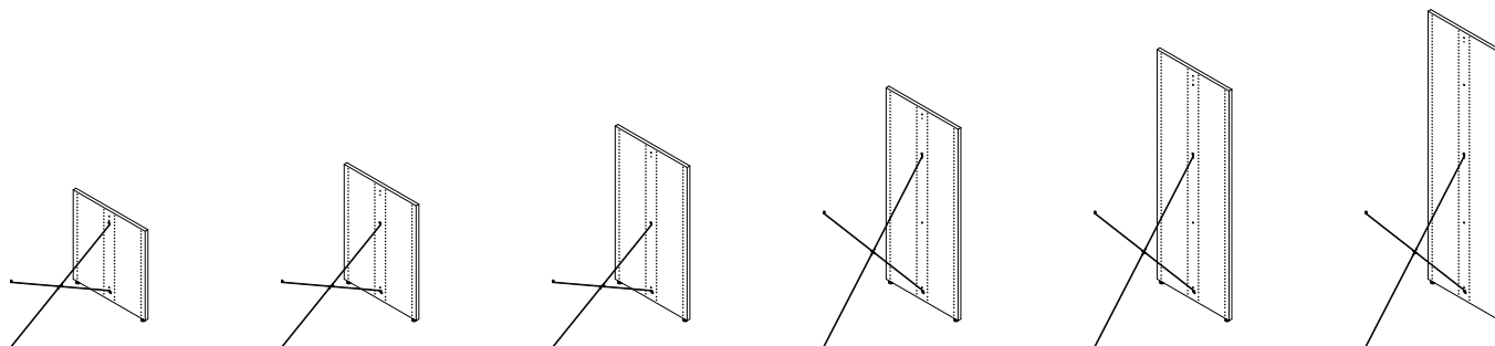
Dubbelsidig mellanstående sektion - H720/920/1220/1520/1820/2120 mm
