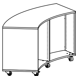
Dubbelsidiga H920 mm - 1/2/3 sektioner
