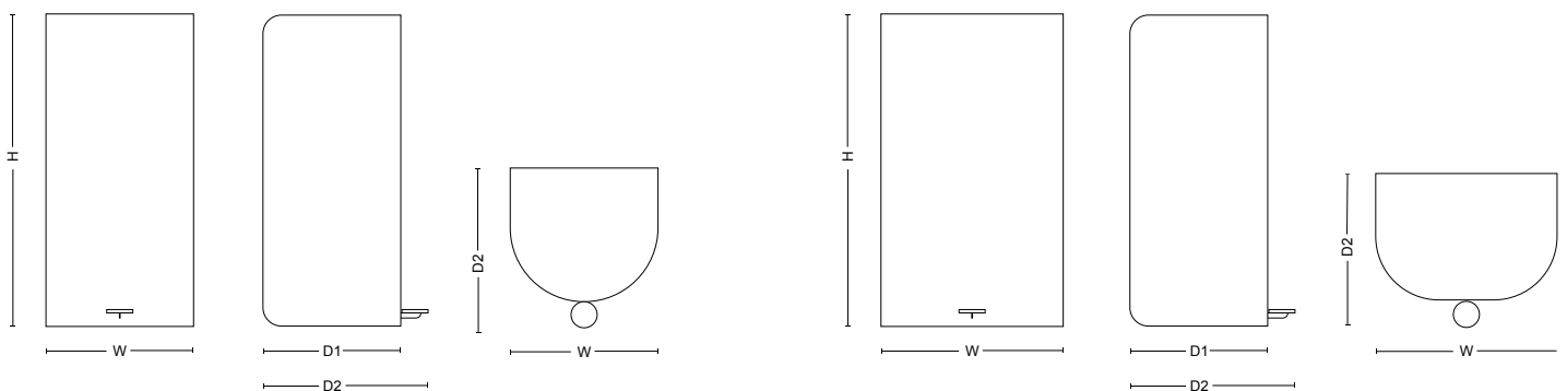
Pelican M H 800 mm, W 360 mm, D1 340 mm, D2 404 Art.nr. 261xx
