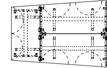
Exempel ihopkoppling av trapetsbord Example of connecting a trapezoidal table
