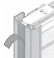
Ⓢ1 U-list med tejp och vinkel. Till modell 3242 levereras vinkel tillsammans med wirefot. Sidolisten kan också monteras på glas.
