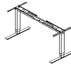
2-parallellsystem, 660 mm slaglängd, 690 mm fötter, teleskoperbar sarg.
