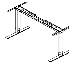
2-parallellsystem, 660 mm slaglängd, 490 mm fötter, teleskoperbar sarg.
