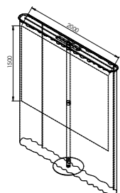
Ljudstopp i akryl för rak Tenda. Höjd 1500 mm. Vajerfästen medföljer.
