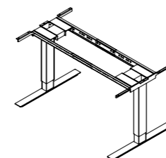
2-parallellsystem med teleskoperbar sarg. 690 mm fötter.
